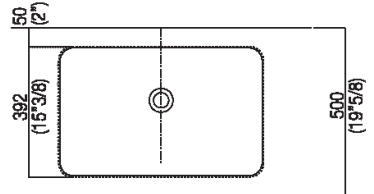
Posizione speciale per rubinetto Sen a parete e Square con bocca curva Special position for wall mounted tap Sen and Square white curved spout
